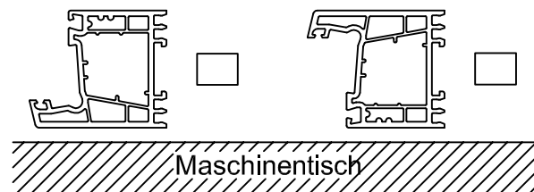
Profilaufgeseite Rahmen
