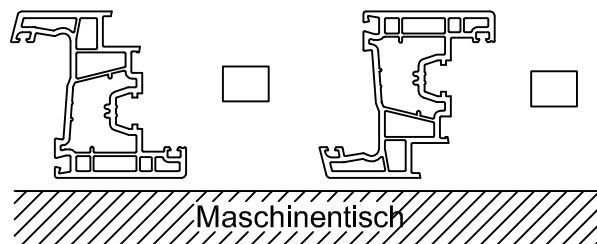
Profilaufgeseite Flügel
